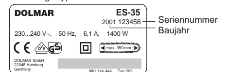
Abbildung: Typenschild ES-35
