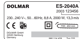
Abbildung: Typenschild ES-2040A
