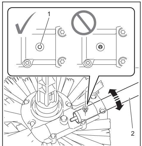
► 1. Hole 2. Pipe
