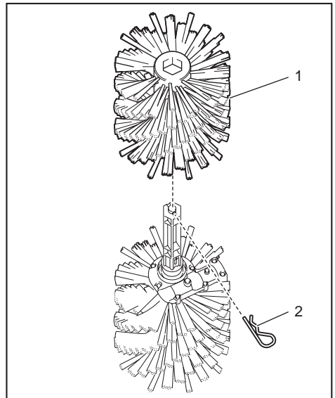
► 1. Spazzolone rotativo 2. Copiglia elastica
