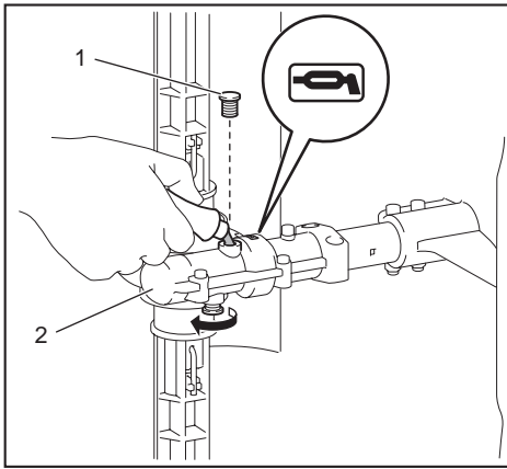
► 1. Bout 2. Tandwielhuis
