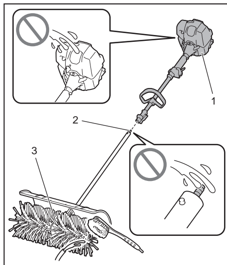
► 1. Aandrijfsysteem 2. Pijpuiteinde 3. Tandwielhuis
