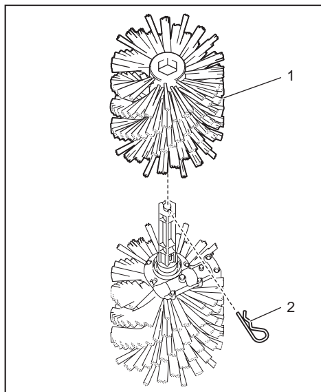
► 1. Bürste 2. Klammer
