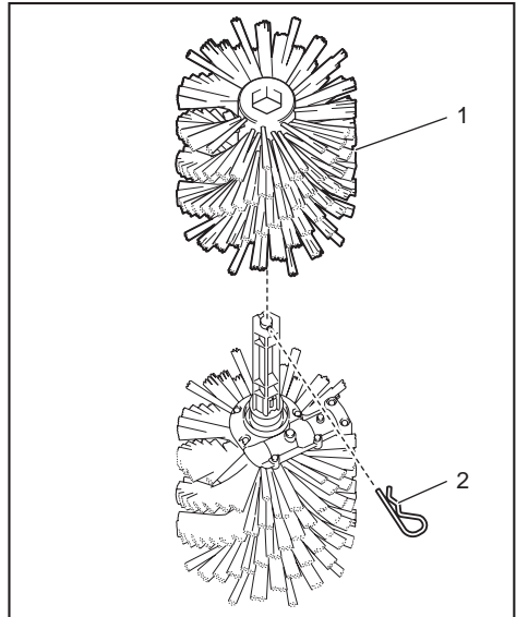
► 1. Brush 2. Clip
