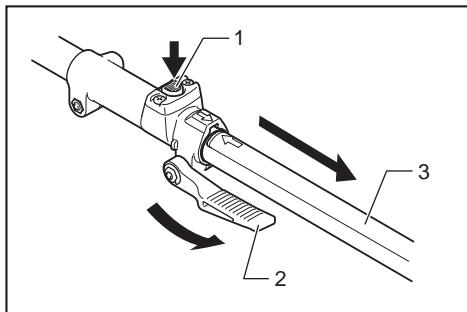
► 1. Botão de libertação 2. Alavanca 3. Tubo
