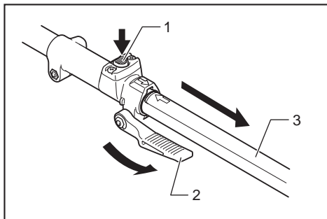
► 1. Pulsante di sblocco 2. Leva 3. Tubo
