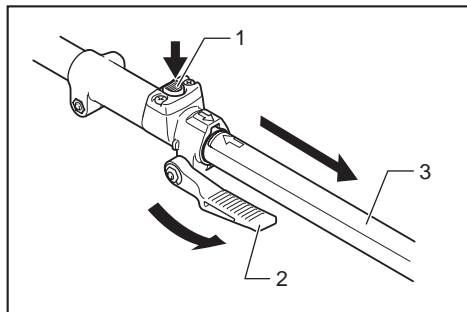
► 1. Udløserknap 2. Håndtag 3. Rør
