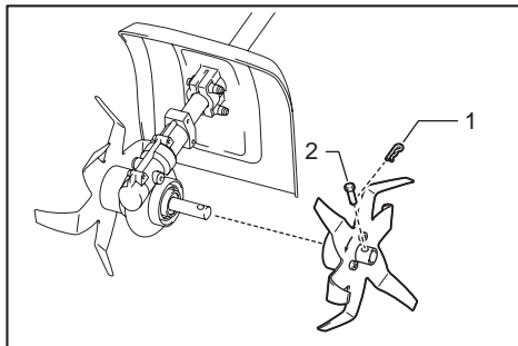
► 1. Klemme 2. Låsestift
