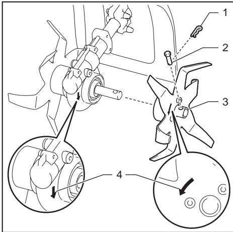
► 1. Grapa 2. Pasador de bloqueo 3. Cubo de la paleta de rotor 4. Marca de flecha
