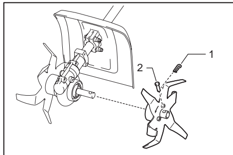
► 1. Graffetta 2. Perno di blocco
