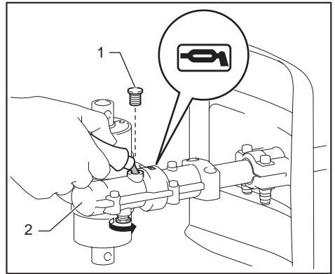
► 1. Perno 2. Caja de engranajes
