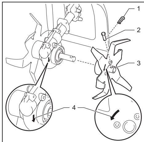
► 1. Graffetta 2. Perno di blocco 3. Mozzo della lama del rotore 4. Simbolo della freccia
