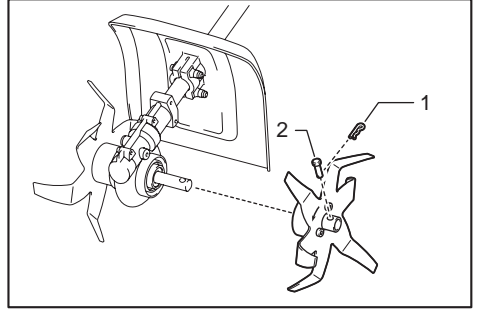
► 1. Klips 2. Kilitleme pimi
