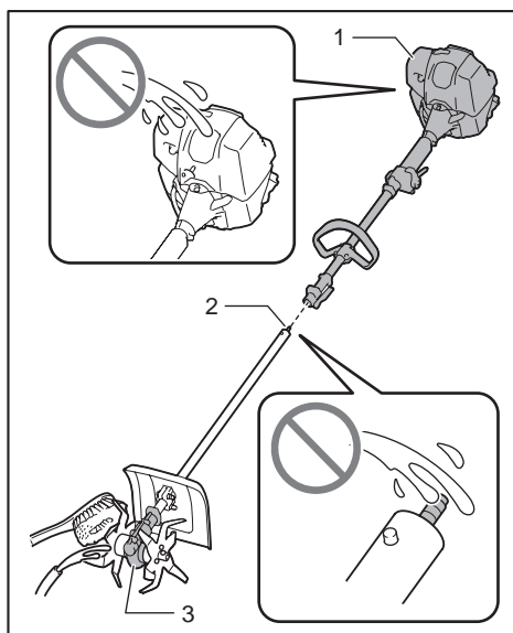
► 1. Outil motorisé 2. Extrémité du tuyau 3. Boîtier d'engrenage
