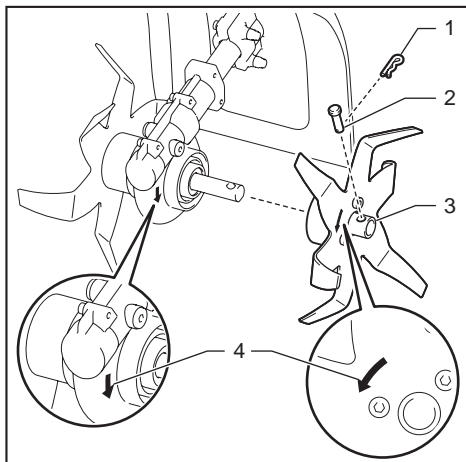
► 1. Klemme 2. Låsestift 3. Nav på den roterende klinge 4. Pilemærke
