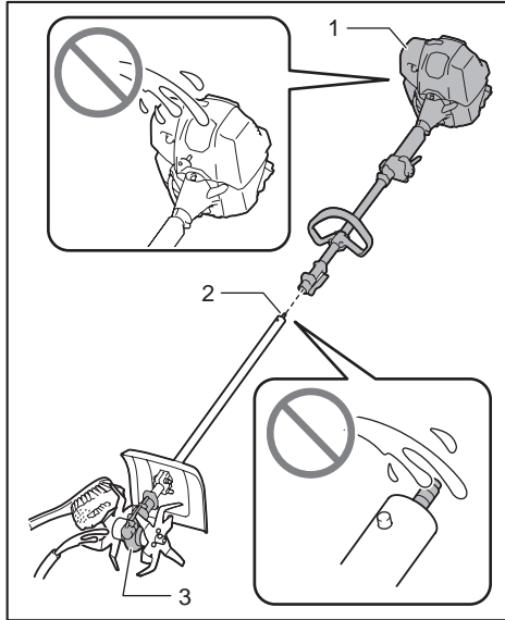
► 1. Μονάδα ισχύος 2. Άκρο σωλήνα 3. Κιβώτιο οδοντωτών τροχών
