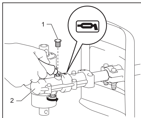
► 1. Bolt 2. Gearhus
