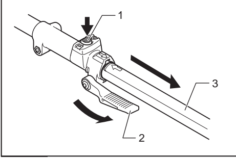
► 1. Serbest bırakma düğmesi 2. Mandal 3. Boru
