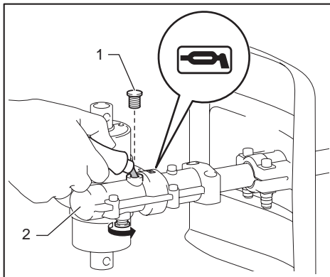
► 1. Schraube 2. Antriebsgehäuse
