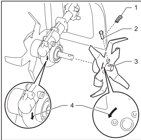
► 1. Klem 2. Borgpen 3. Naaf van het rotormes 4. Pijlmarkering
