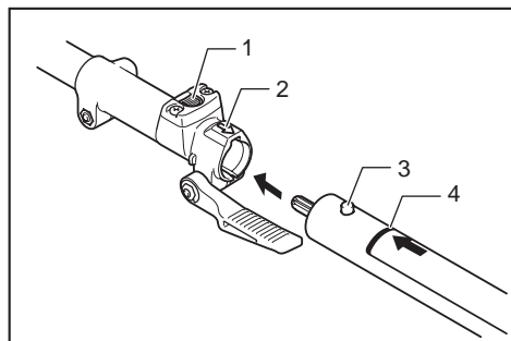
► 1. Pulsante di sblocco 2. Simbolo della freccia 3. Perno 4. Linea di posizione
