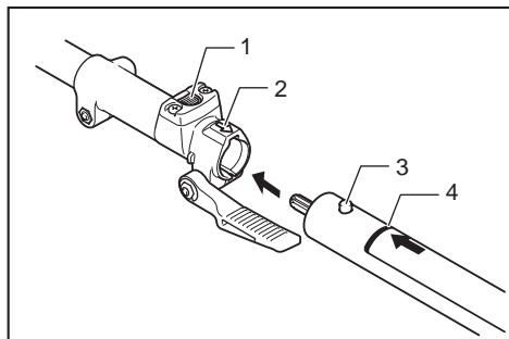
► 1. Botão de libertação 2. Marca da seta 3. Pino 4. Linha de posição
