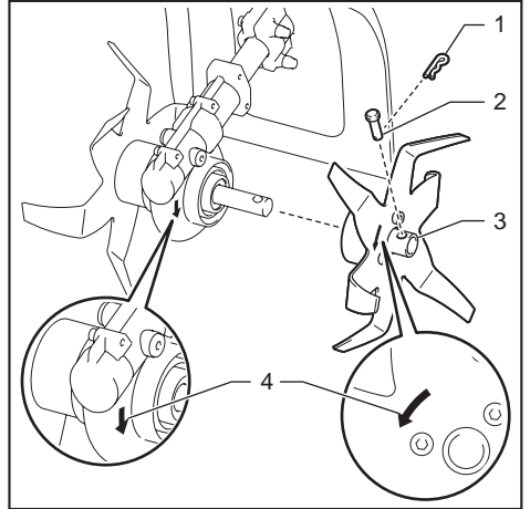
► 1. Klips 2. Kilitleme pimi 3. Rotor bıçağı göbeği 4. Ok işareti
