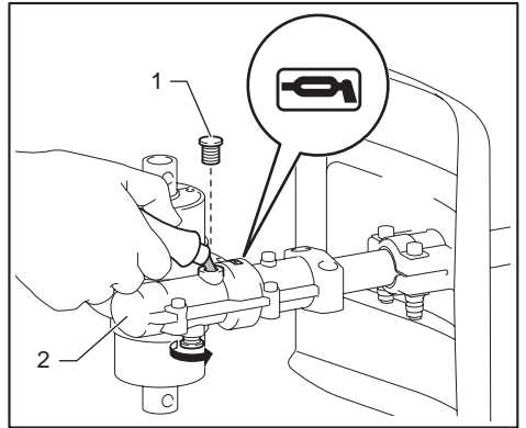
► 1. Bout 2. Tandwielhuis
