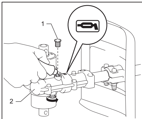
► 1. Bullone 2. Scatola degli ingranaggi
