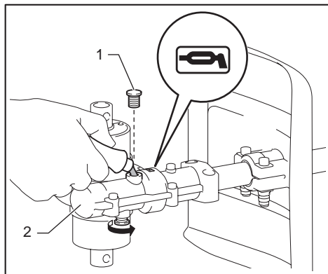
► 1. Μπουλόνι 2. Κιβώτιο οδοντωτών τροχών
