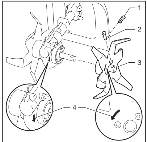
► 1. Κλιπ 2. Πείρος ασφάλισης 3. Κέντρο στήριξης της λάμας ρότορα 4. Σημάδι βέλους
