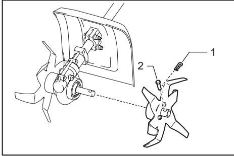
► 1. Grapa 2. Pasador de bloqueo
