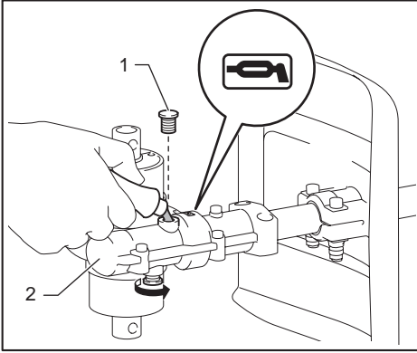
► 1. Civata 2. Dişli kutusu
