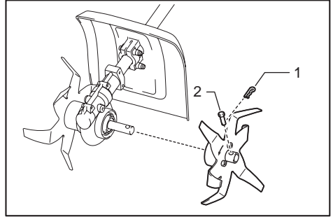
► 1. Κλιπ 2. Πείρος ασφάλισης
