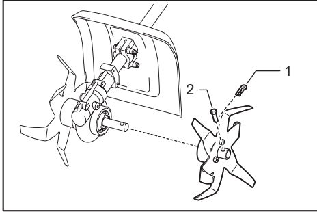
► 1. Klem 2. Borgpen
