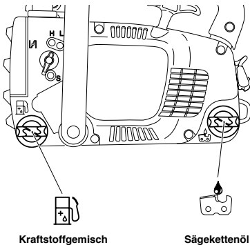
Kraftstoffgemisch
