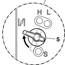
Κρύα εκκίνηση
