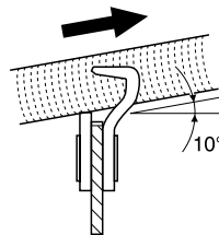
Τύπος αλυσίδας 492, 466
