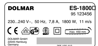
Abbildung: Typenschild ES-1800
